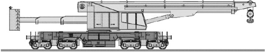
Bild 4 Fahrzeugkran: Schienenkran mit Seilwinde
